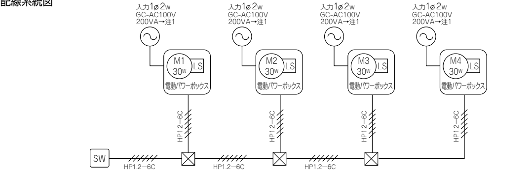
配線系統図
