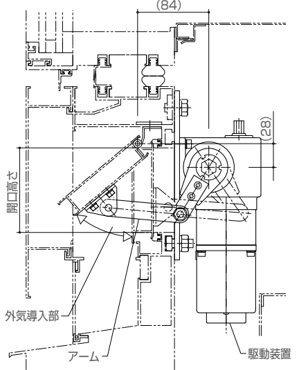
縦断面図
