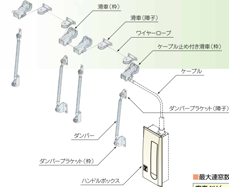
※上図は外倒し窓(MD-W)納まり
