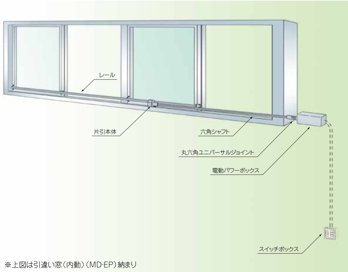
配線系統図 (排煙仕様)
