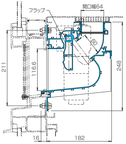
縦断面図
