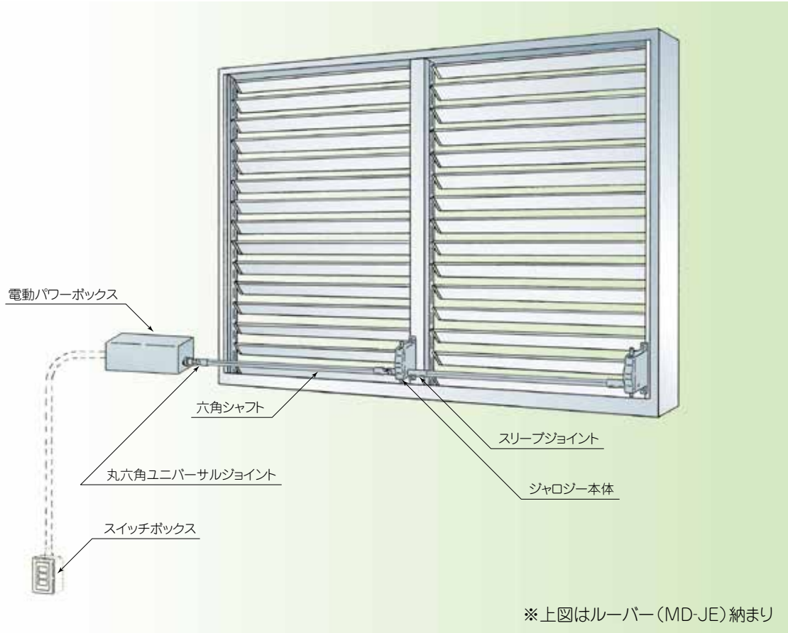
配線系統図
