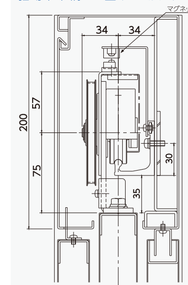
駆動吊車納まり図 (レール標準型)
