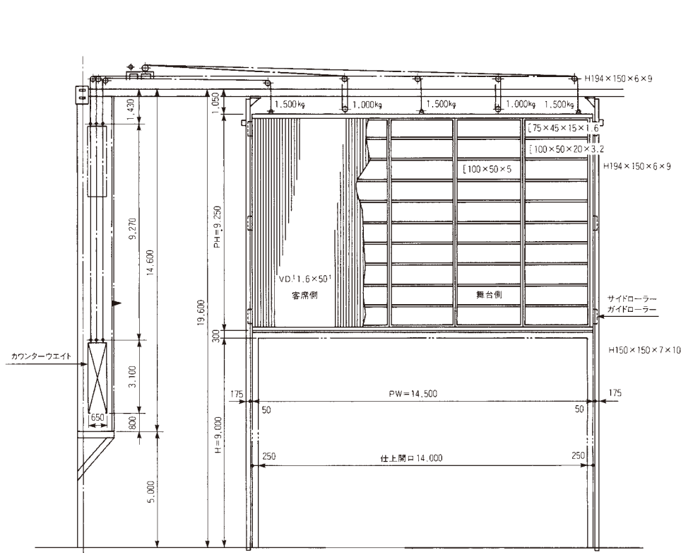
納まり図
