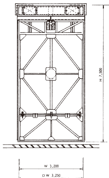
■中折れドア前面図
