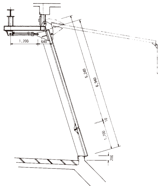
■中折れドア側面図
